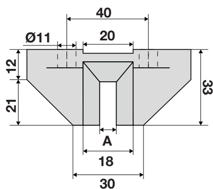
PATTINO CONTRAPPESO QUADRO
