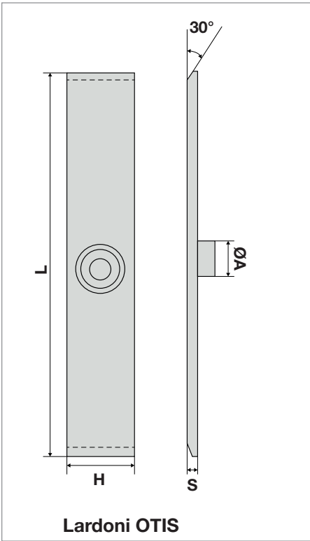
Pattino guida FALCONI L.158
