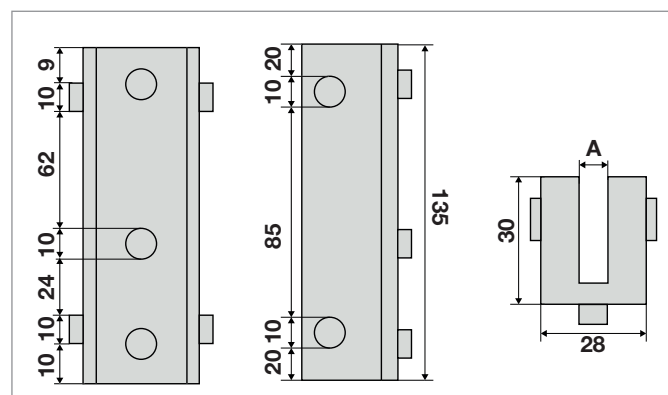
Pattino L.135 SCHINDLER
