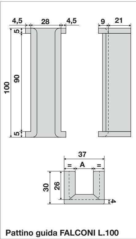
Pattino guida FALCONI L.100
