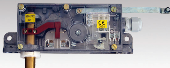
ELF 1 e EL 1 (EN 81-21)
