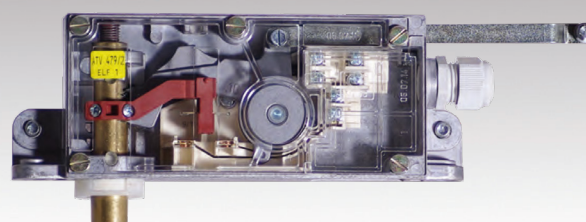
ELF 1 e EL 1
